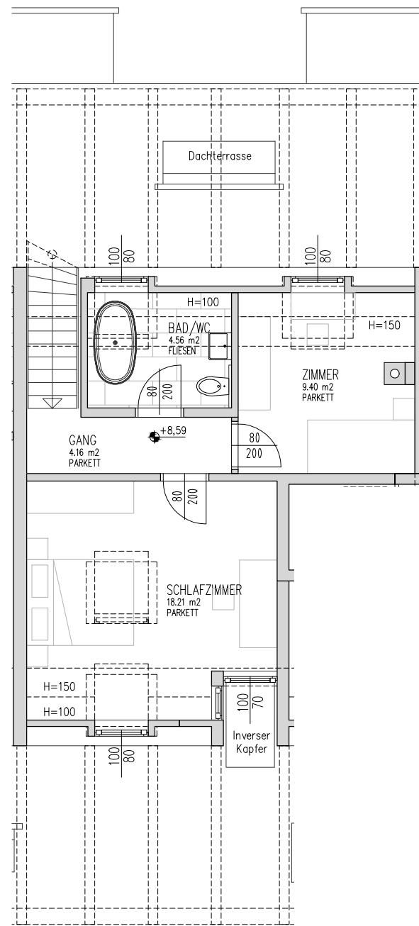
DACHGESCHOSS 2
